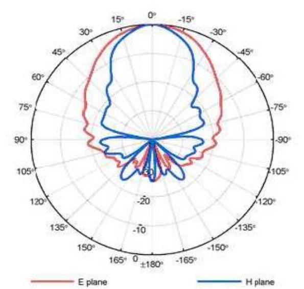
Typ. 3GHz Pattern
