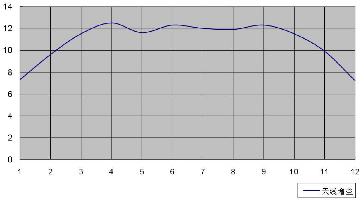
天线增益
