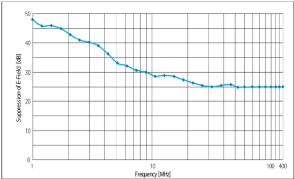
E-Field Suppression
