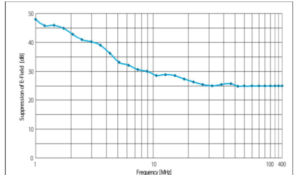
E-Field Suppression
