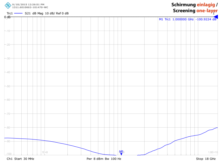
Schirmung einlagig / Screening one-layer
