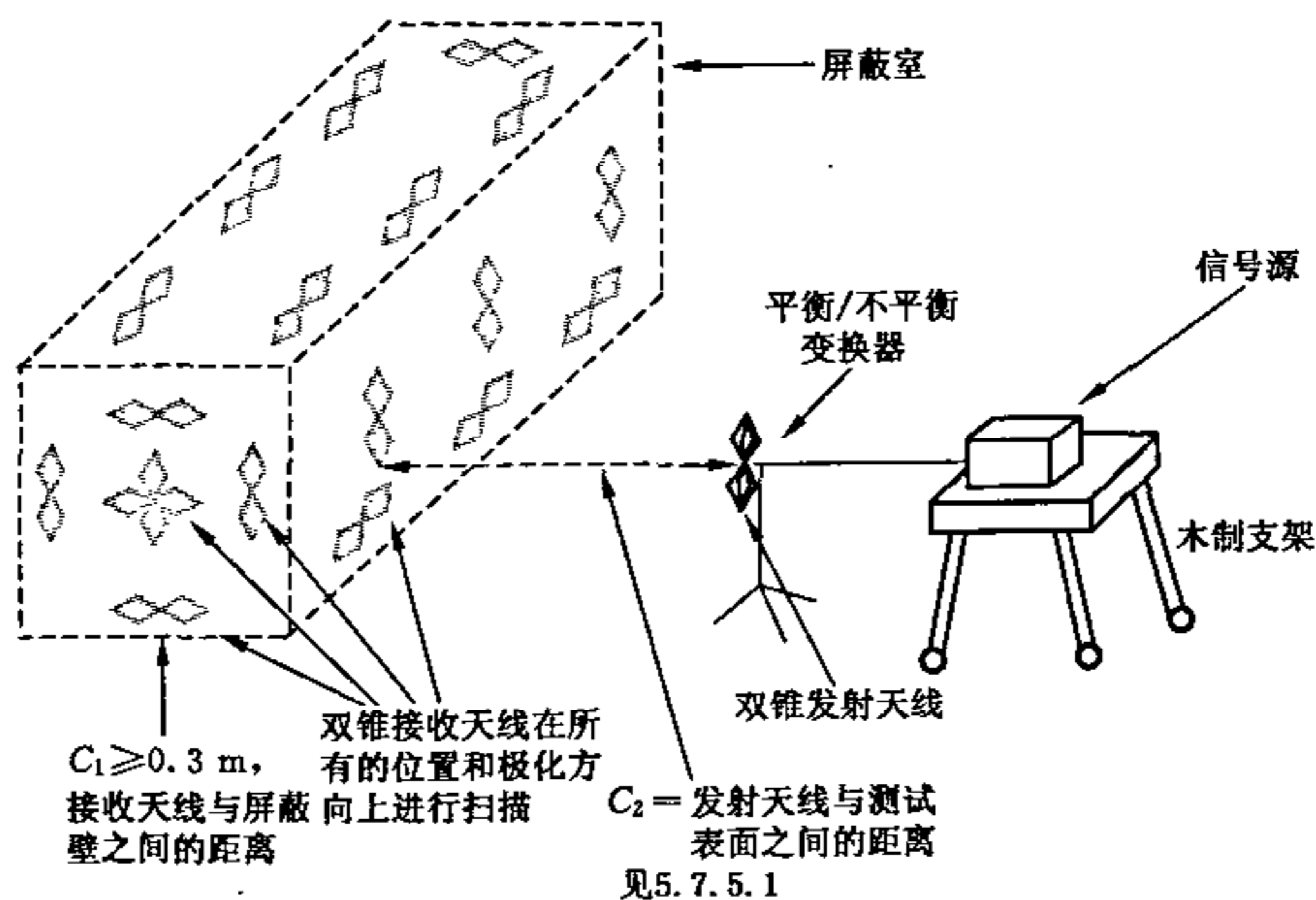
a) 谐振范围测量布置(发射天线水平极化), 20 MHz~100 MHz
