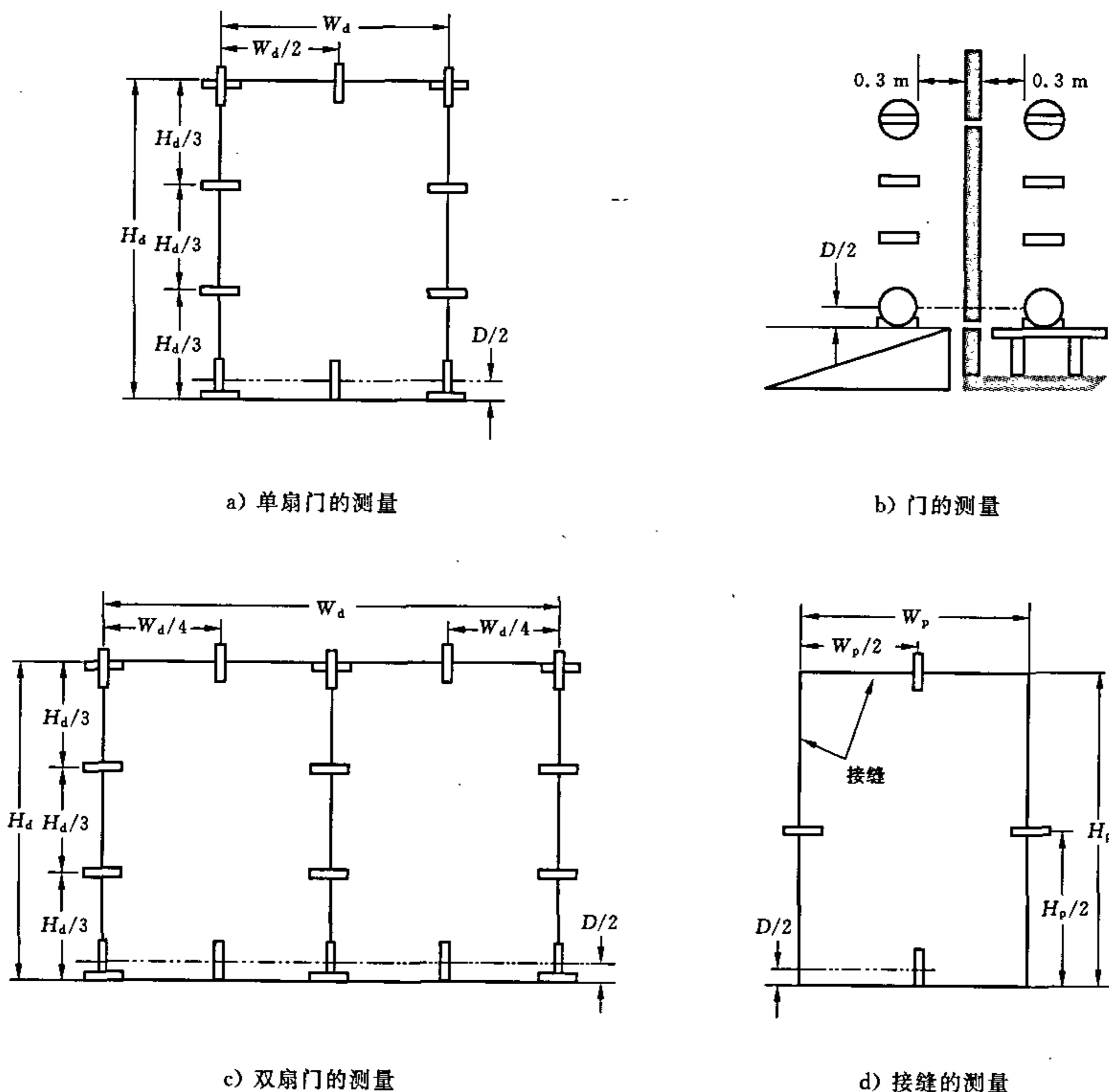
图 2 低频测试中环天线的标准位置
