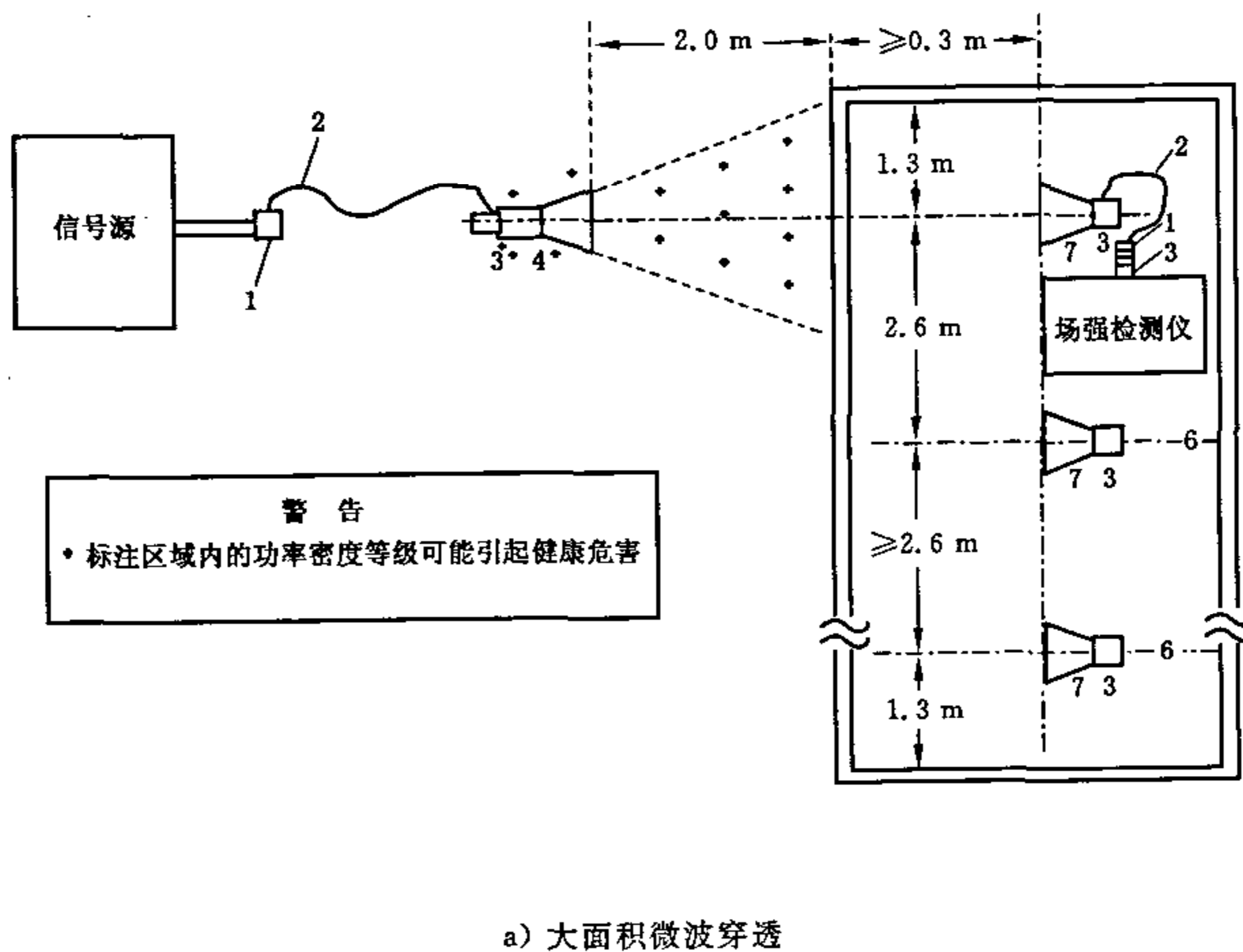
图 8 参考和测量配置(频率高于 1 GHz)
