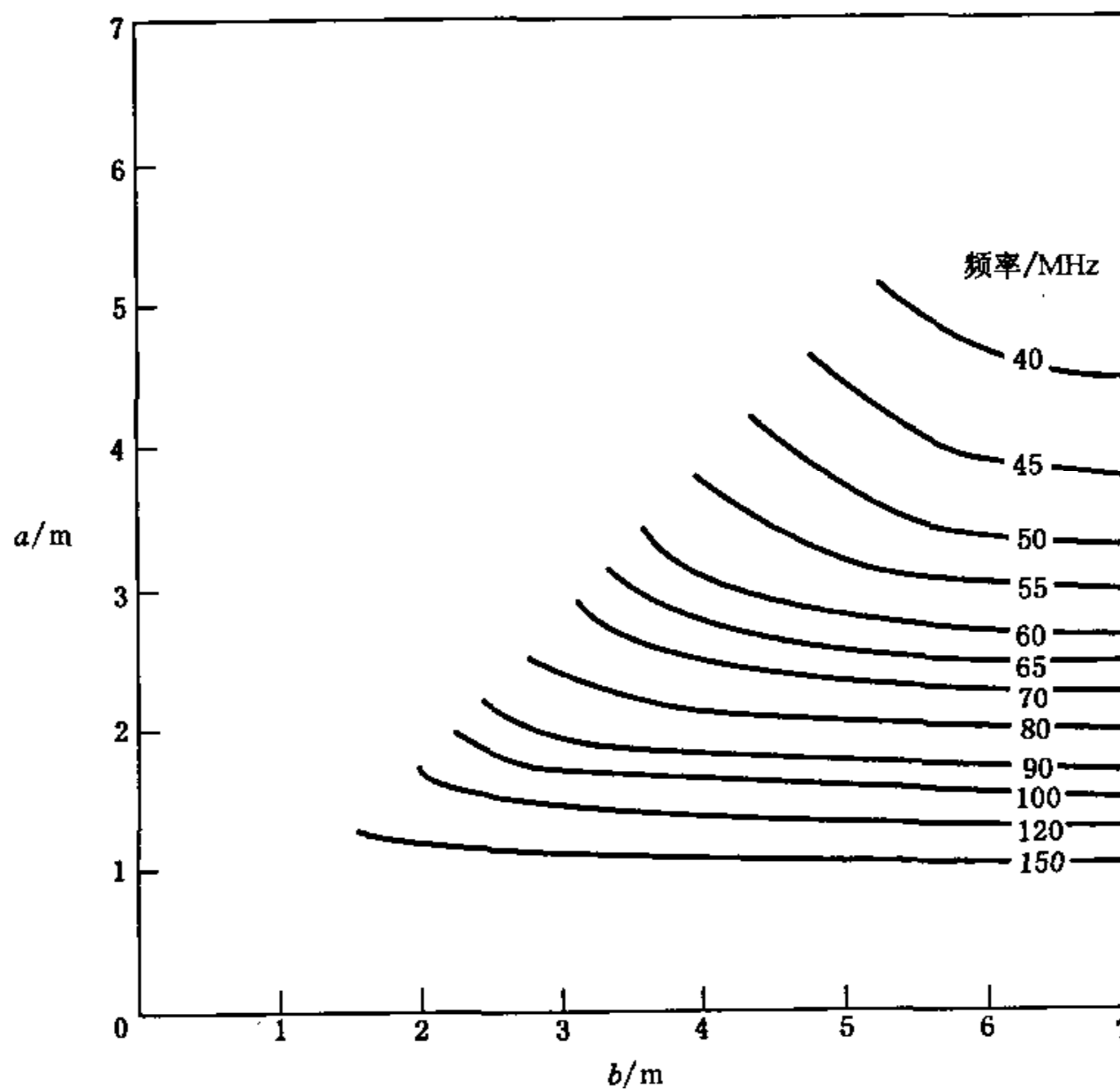
图 5 最低固有谐振频率图
