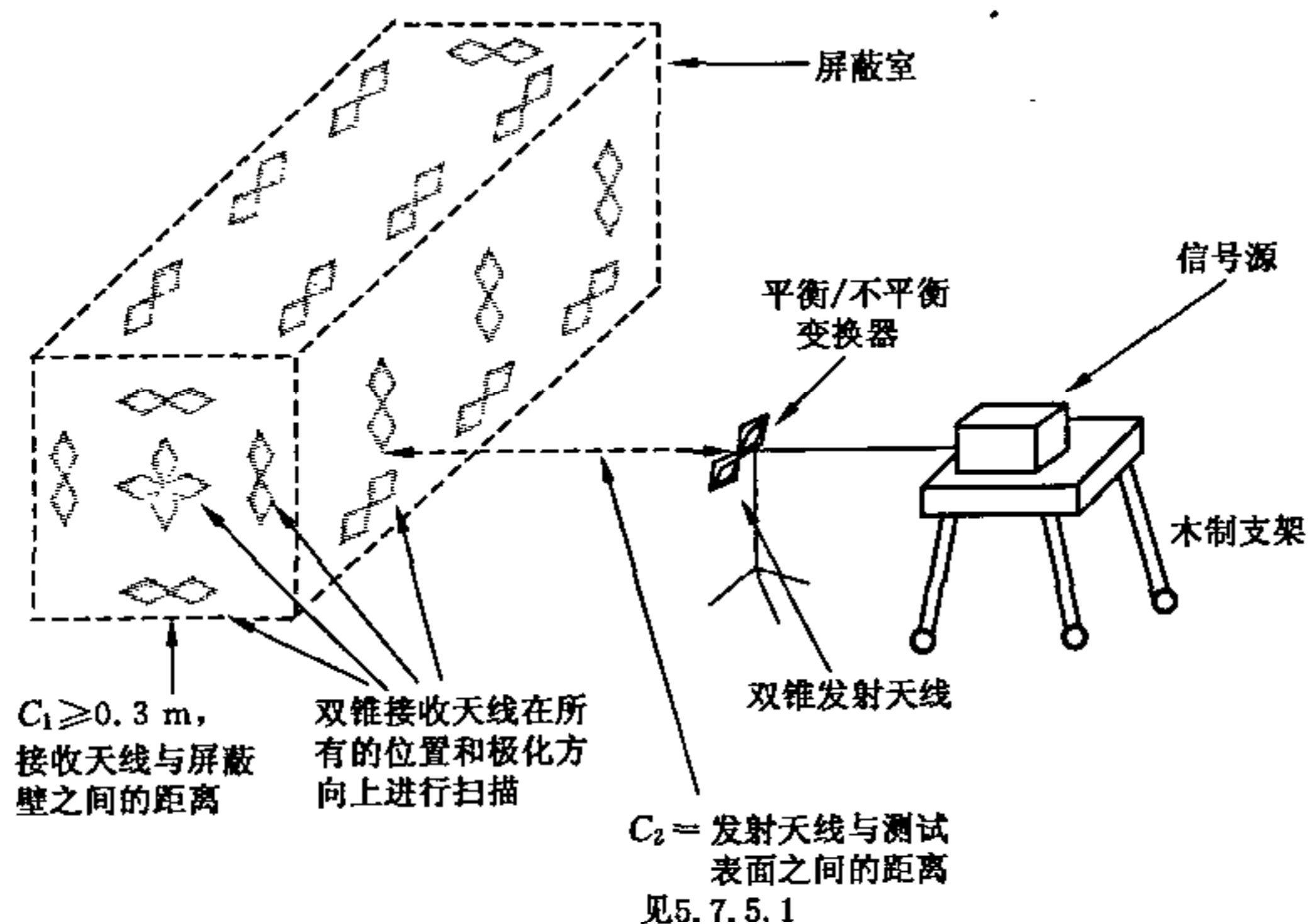
a) 谐振范围测量布置(发射天线水平极化), 20 MHz~100 MHz
