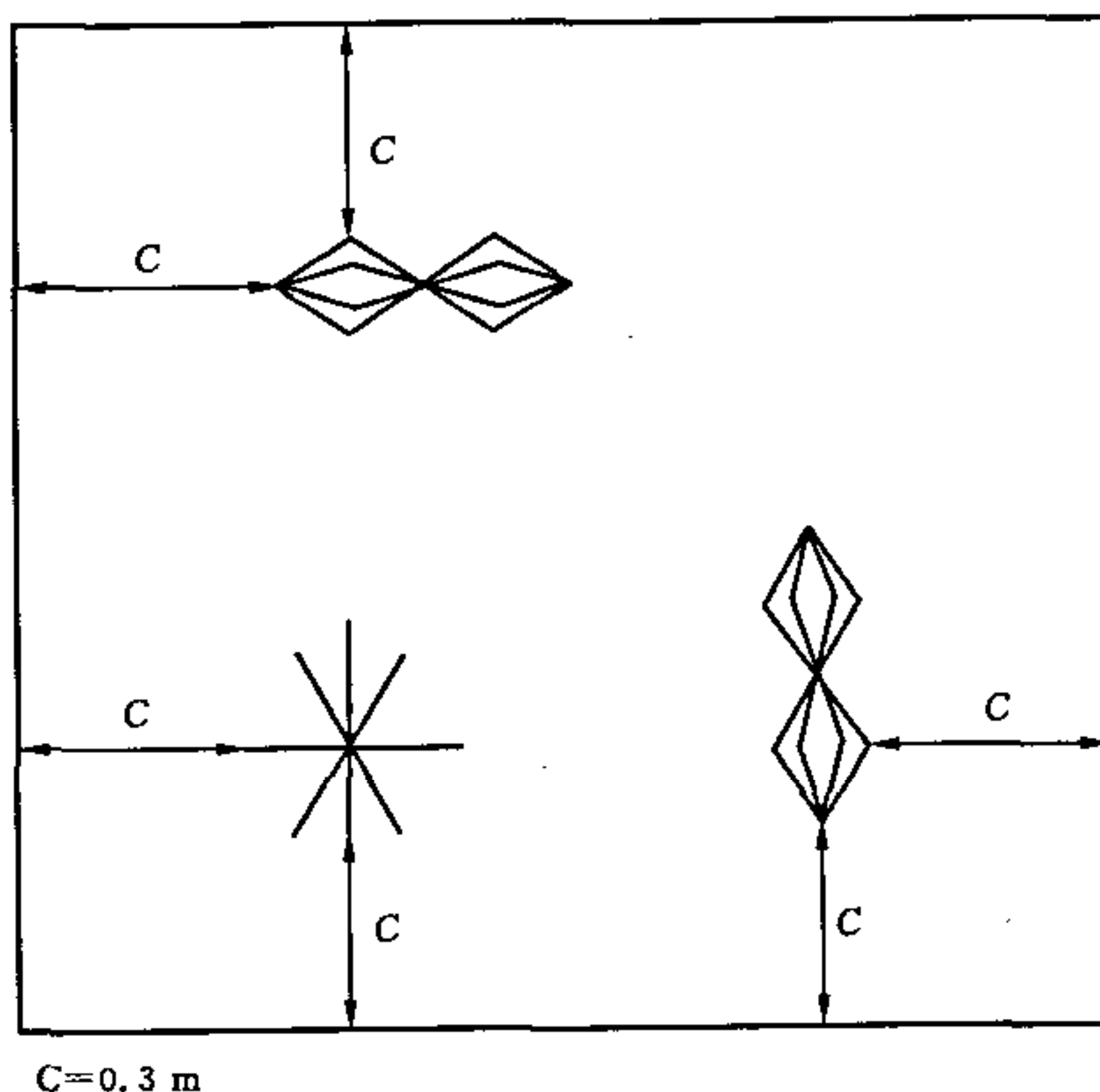
图 A.1 天线到屏蔽墙体的最小距离
