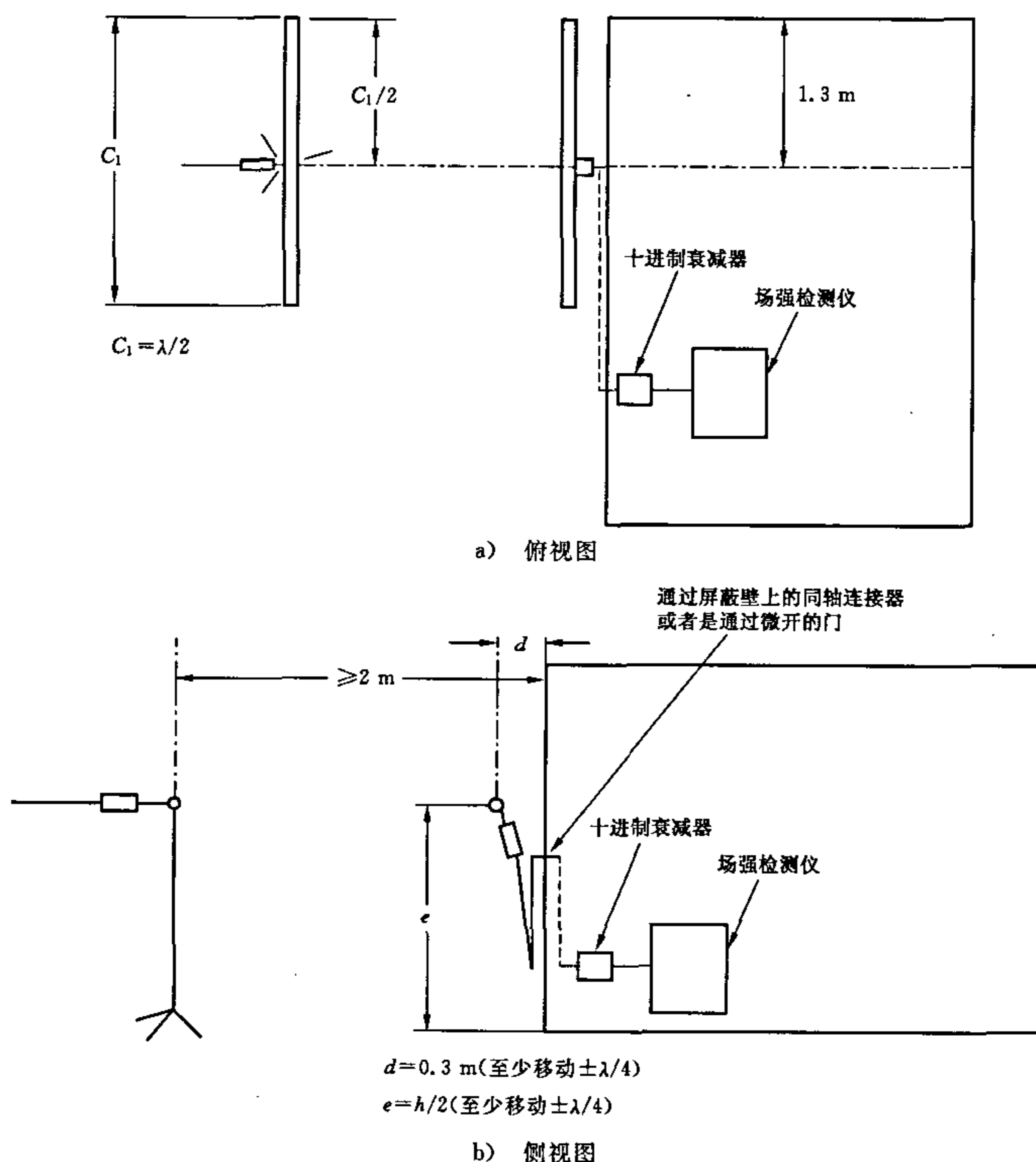
图 6 参考测量配置(频率低于 1 000 MHz)
