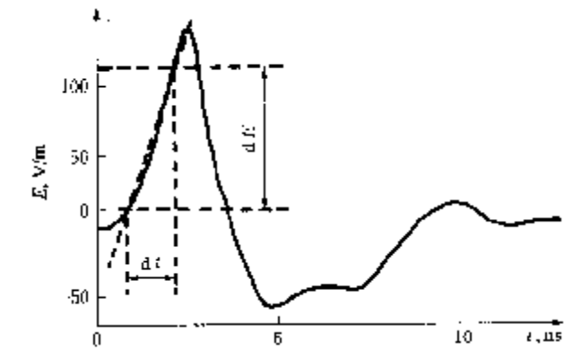
图 C2 距静电放电 1 m 处的电场
