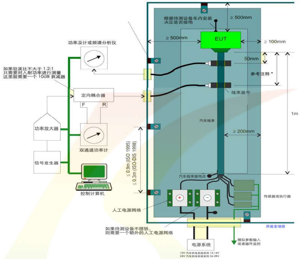
ISO11452-4 大电流注入系统配置图
