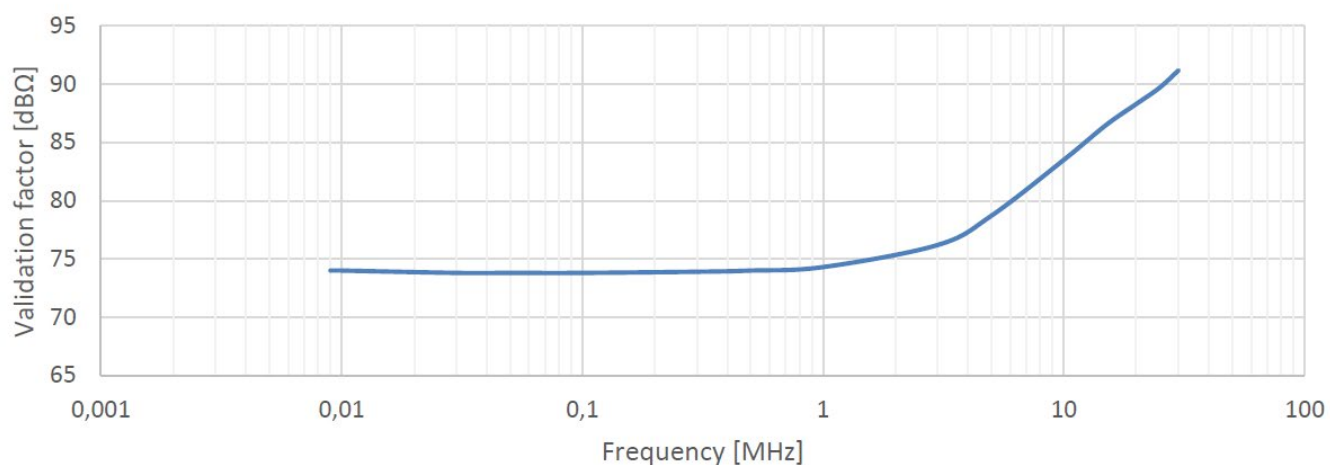
CISPR 16-1-4 验证因子
